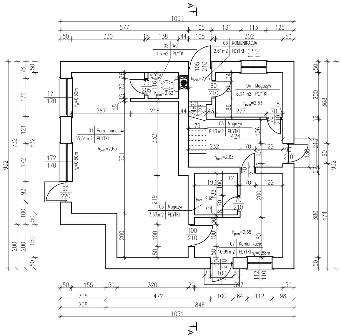
RZUT PRZYZIEMIA skala 1:50
